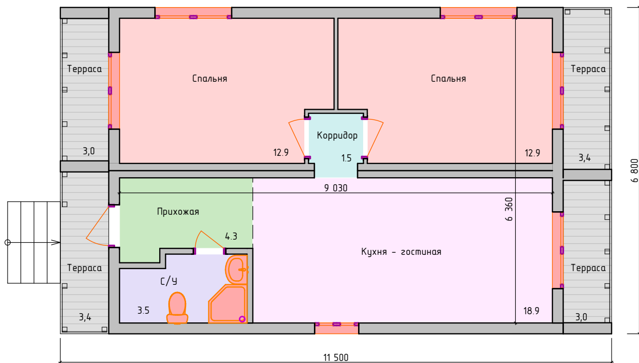
План дома
